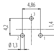
Bohrbilder Buchseneinsatz (Leiterplatte), ungeschirmt Drilling schemes female insert (PCB), unshielded
